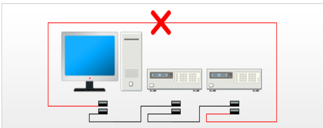
Рисунок 4. Внимание: устройства не должны быть подключены последовательно.
