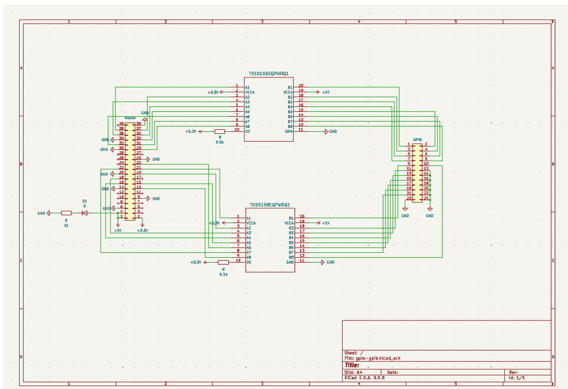
Рисунок 5 — Структурная схема контроллера GPIO–GPIB на базе Repka Pi 3
