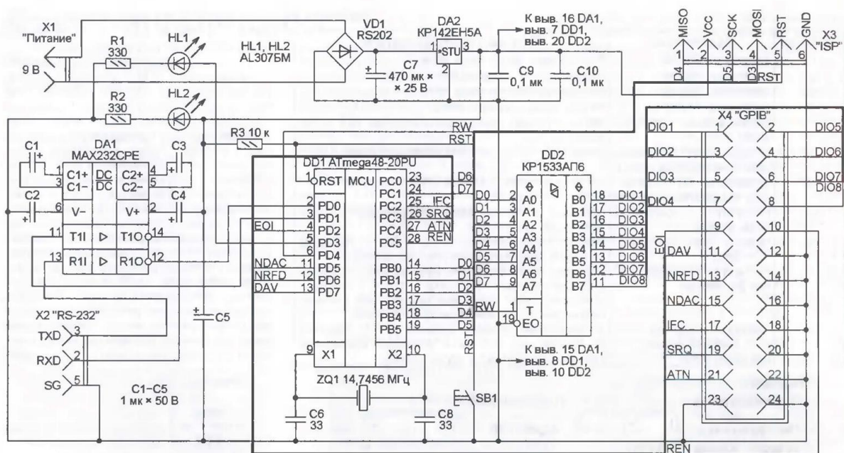
Рисунок 9 — Схема контроллера GPIB из журнала «Радио»
