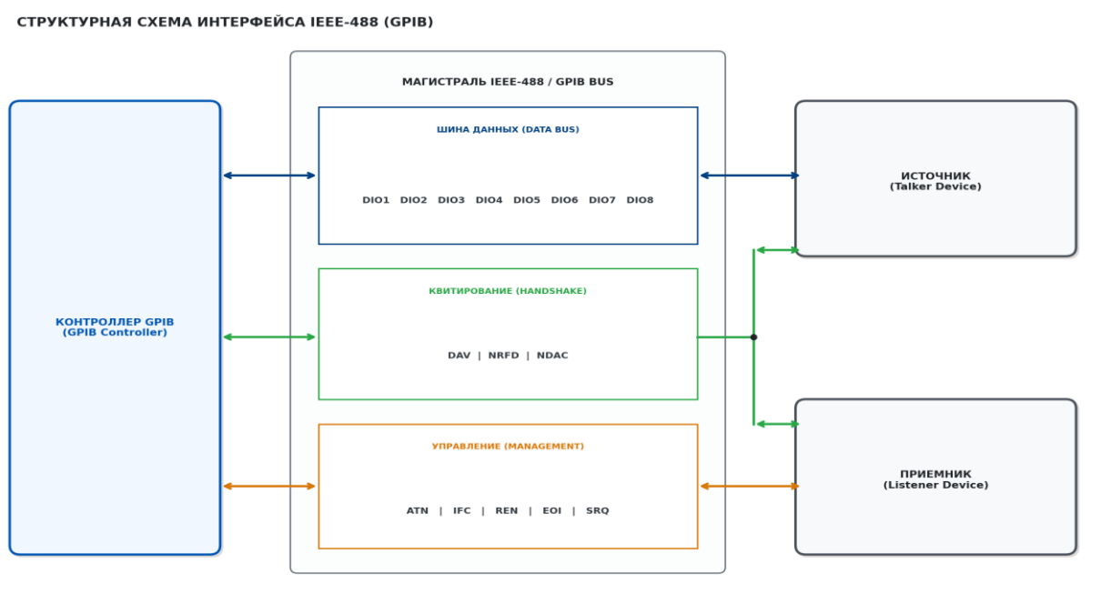
Рисунок 1 — Общая структура интерфейса IEEE-488 (GPIB)
