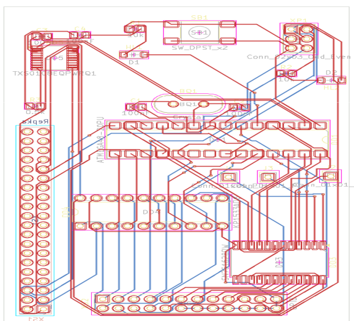
Рисунок 12 — Печатная плата UART–GPIB контроллера
